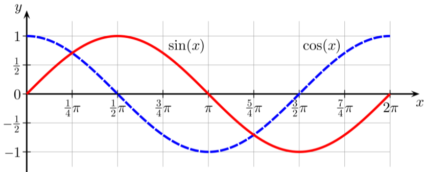
Abb. 3: SINUS und COSINUS-Graph der Funktionen \sin(x) und \cos(x) . Eine Periode von 0 bis 2\pi ist dargestellt. Die x-Achse ist in \pi -Anteilen skaliert entsprechend 0 bis 2\pi bzw. 0^\circ bis 360^\circ
